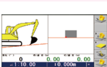
バックホウへ取付するモニタ画面(表示例)
