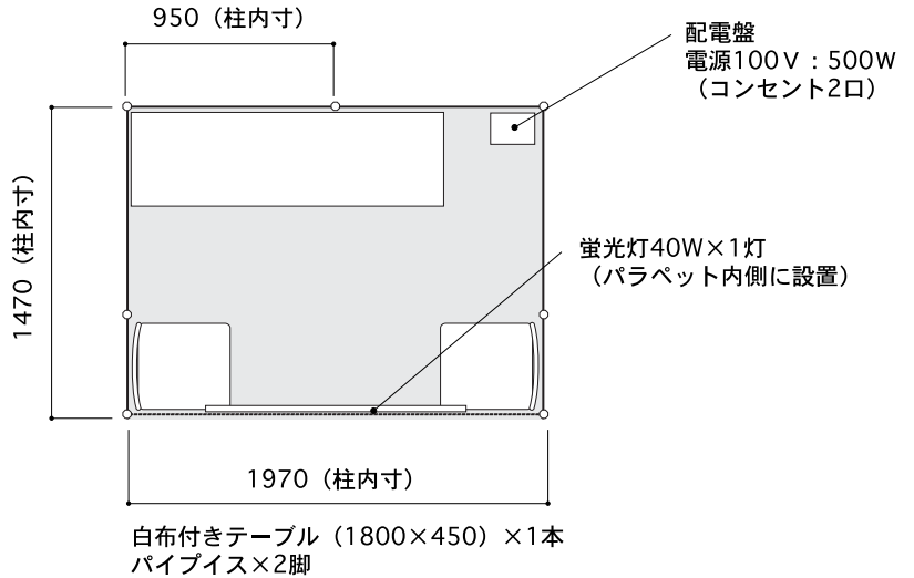
□平面図
